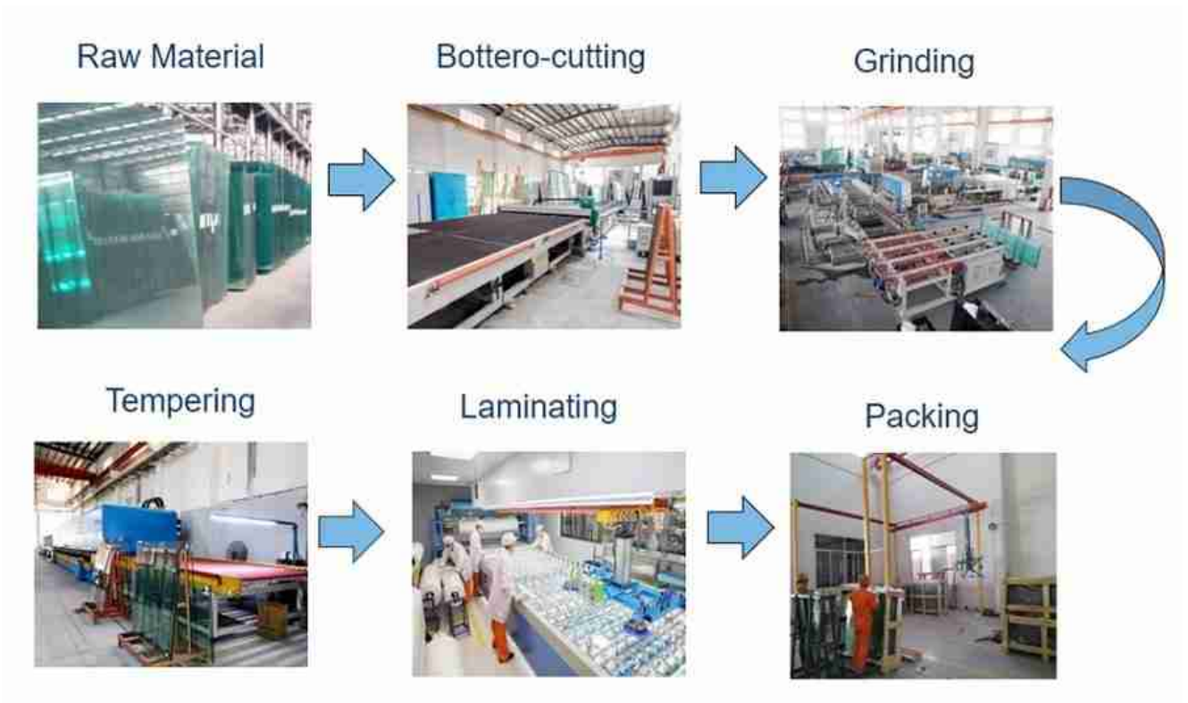
quy trình sản xuất kính âm thanh nhiều lớp
