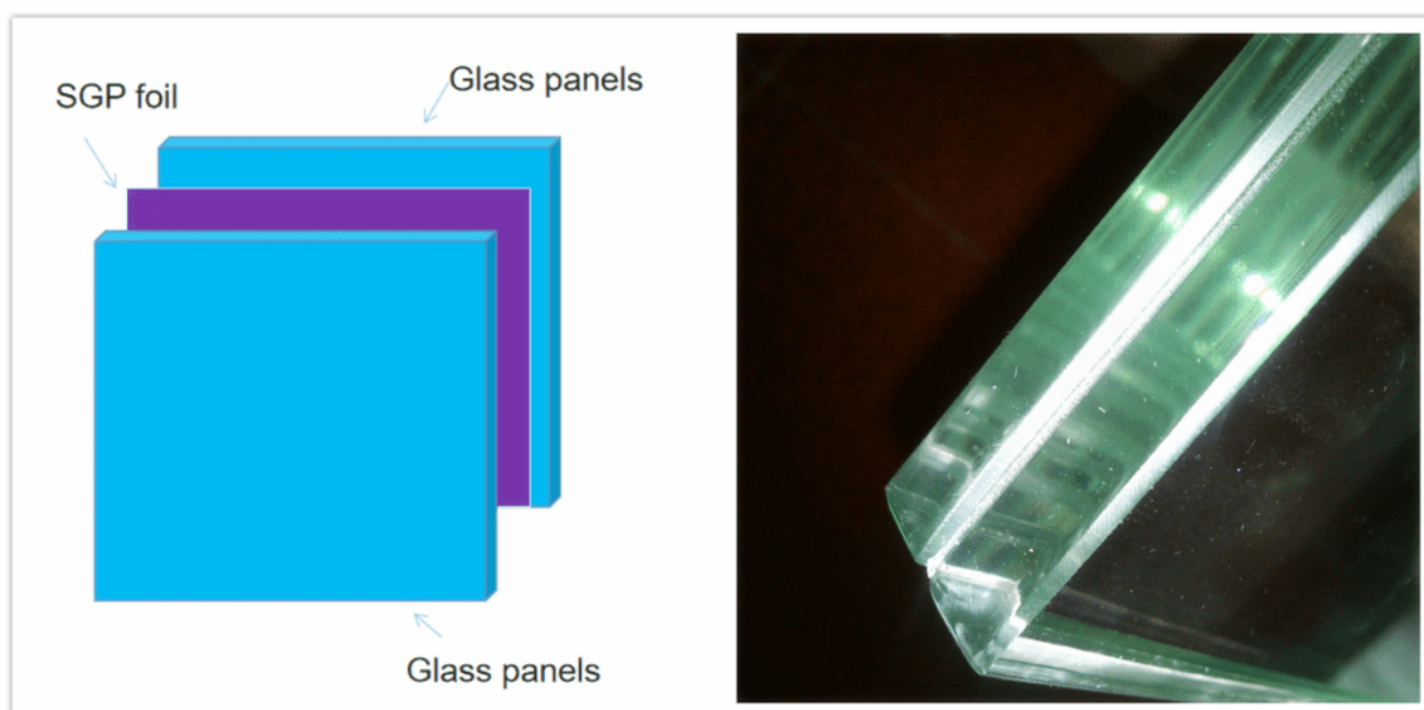
Структура ламинированного стекла
