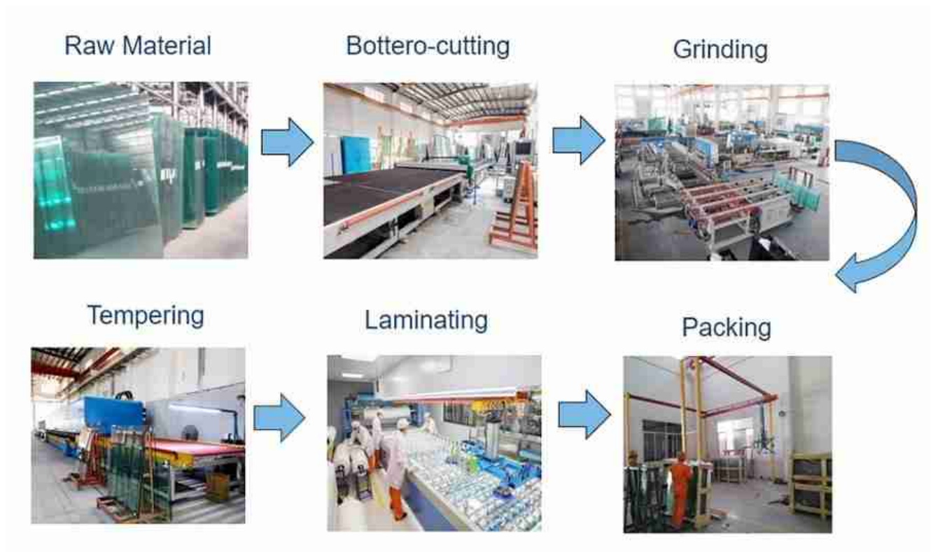
laminert akustisk glassproduksjonsprosess
