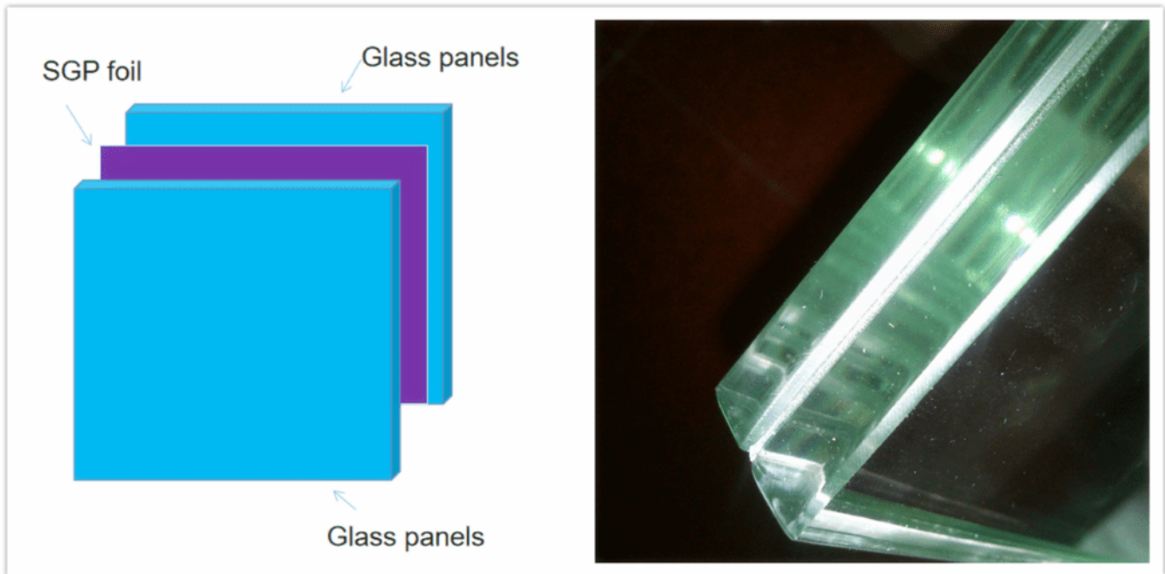
Laminierte Glasstruktur
